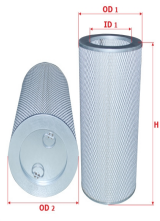
A-87660 ES-12458
