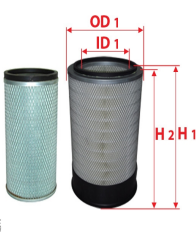
A-87640-S ES-12456
